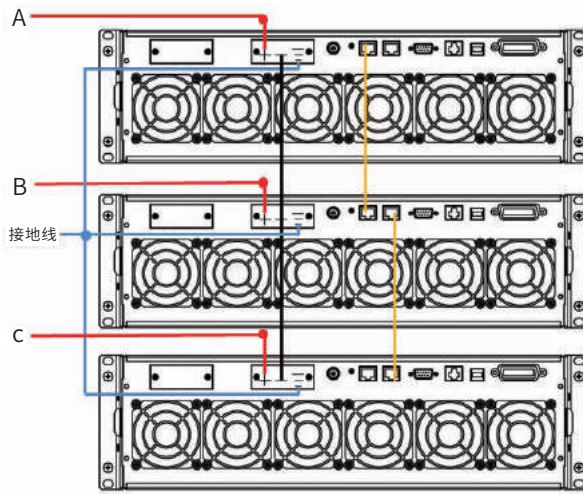
三角形接法
