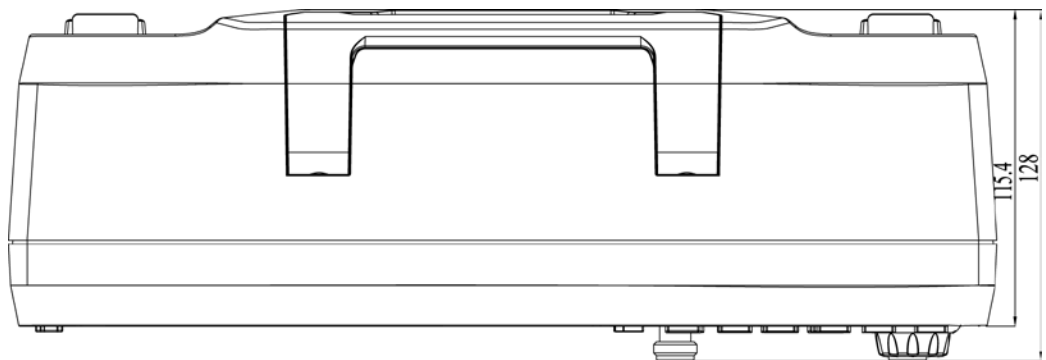
图 1-2 侧视图
