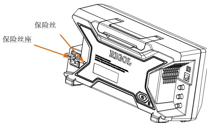
图 1-16 更换保险丝
