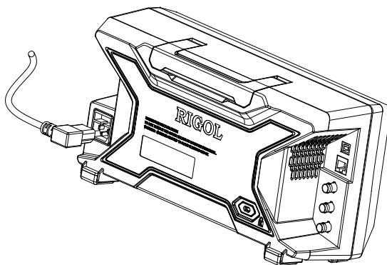
图 1-4 连接电源线
