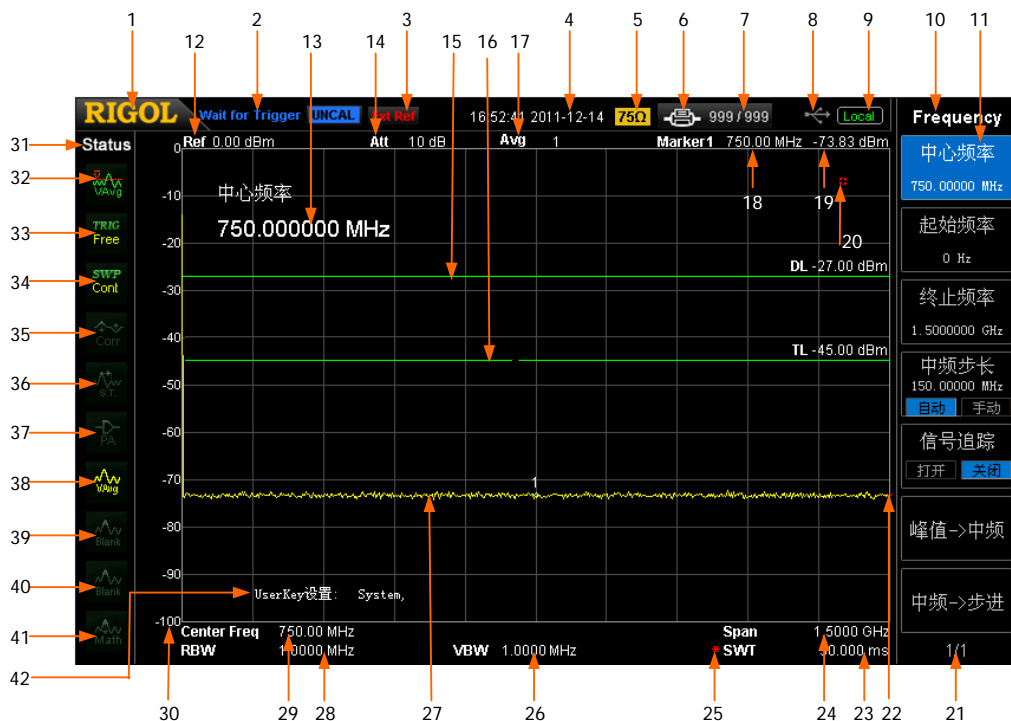
图 1-10 用户界面
