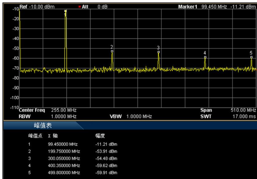
图 2-26 峰值表
