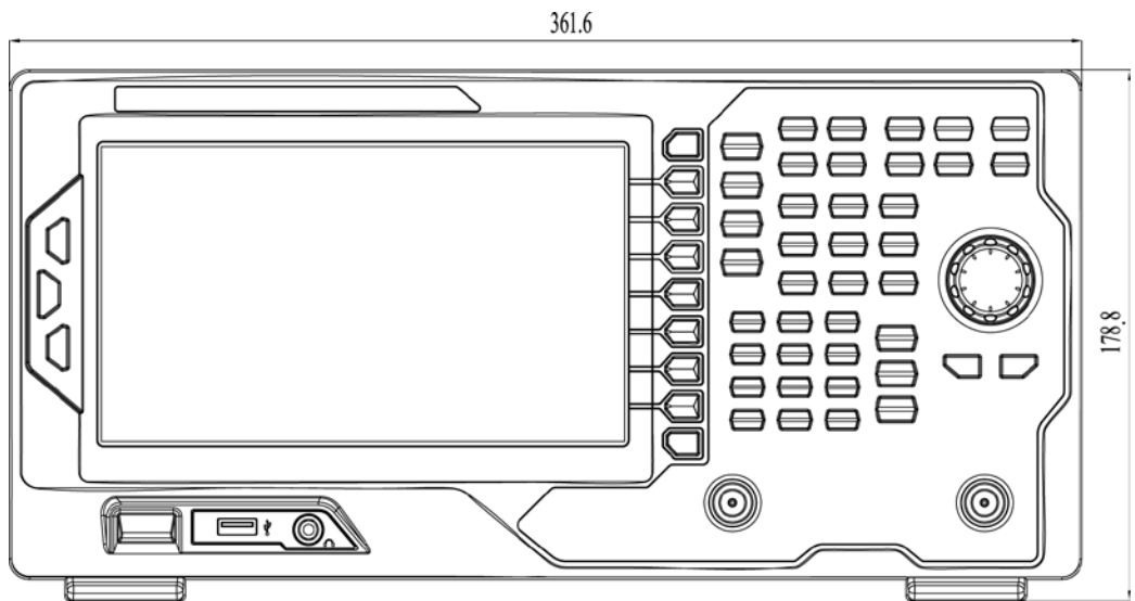
图 1-1 正视图
