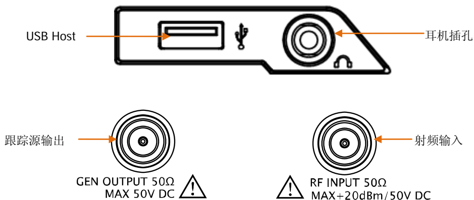
图 1-7 前面板连接器
