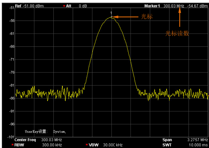
图 2-22 光标示意图
