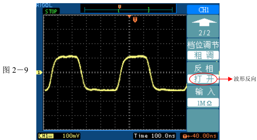
反相的波形
