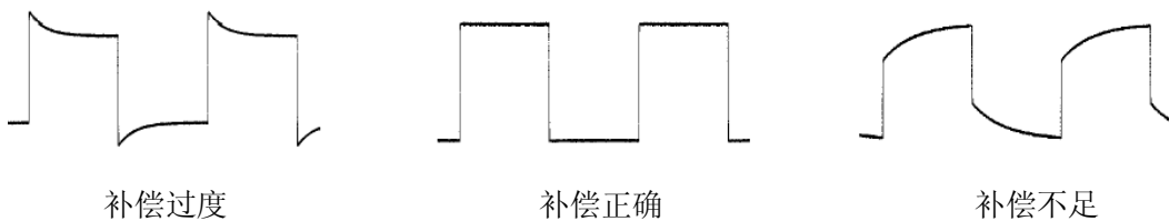
图 1-9 探头补偿
