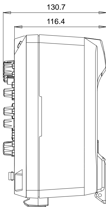
图 1-2 侧视图
