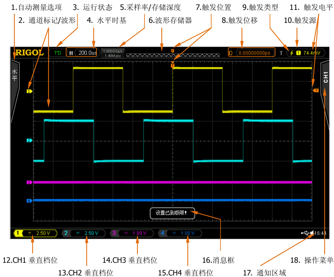
图 1-12 用户界面
