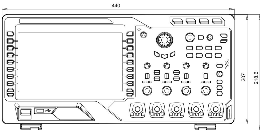
图 1-1 正视图
