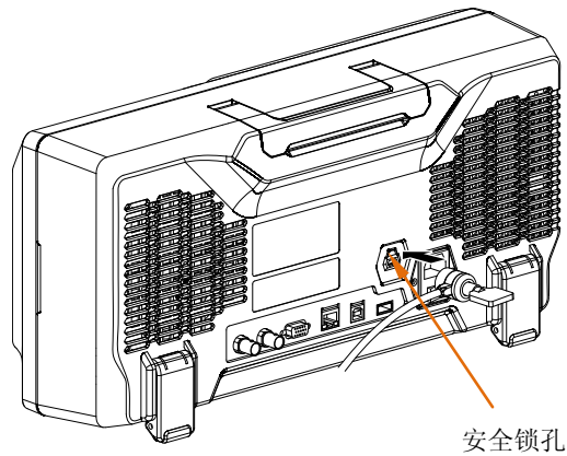
图 1-13 使用安全锁
