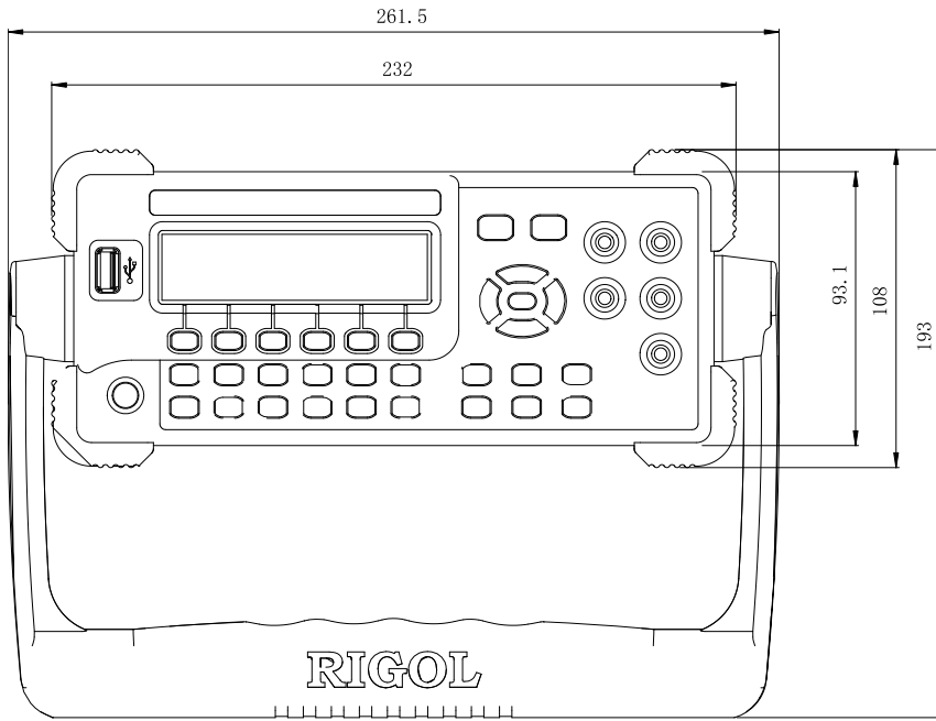
图 1-3 正视图
