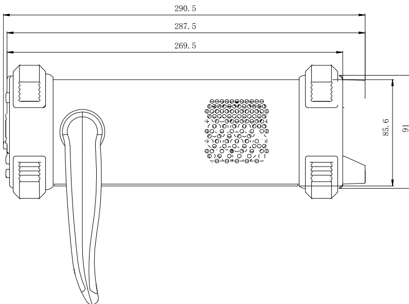
图 1-4 侧视图
